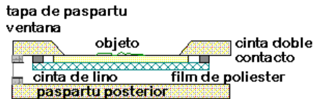
Sistema de paspartu carpeta para documentos con superficies sensibles, y texto en el reverso
