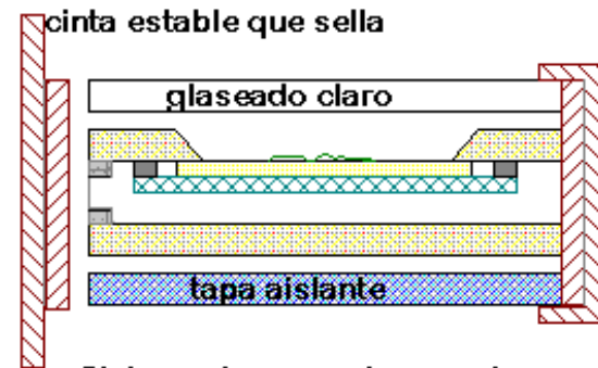
Sistema de paspartu carpeta tipo "paquete sellado"
